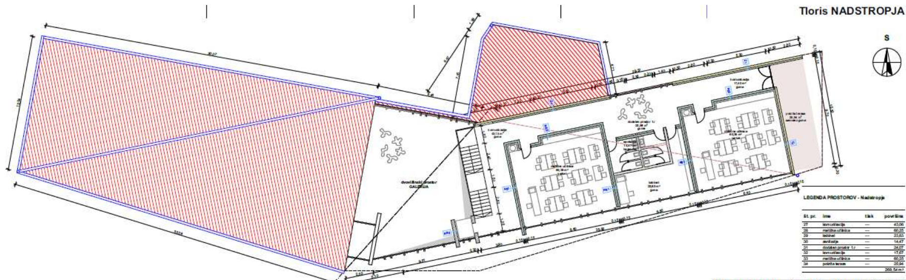
Slika 2: Tloris nadstropja
