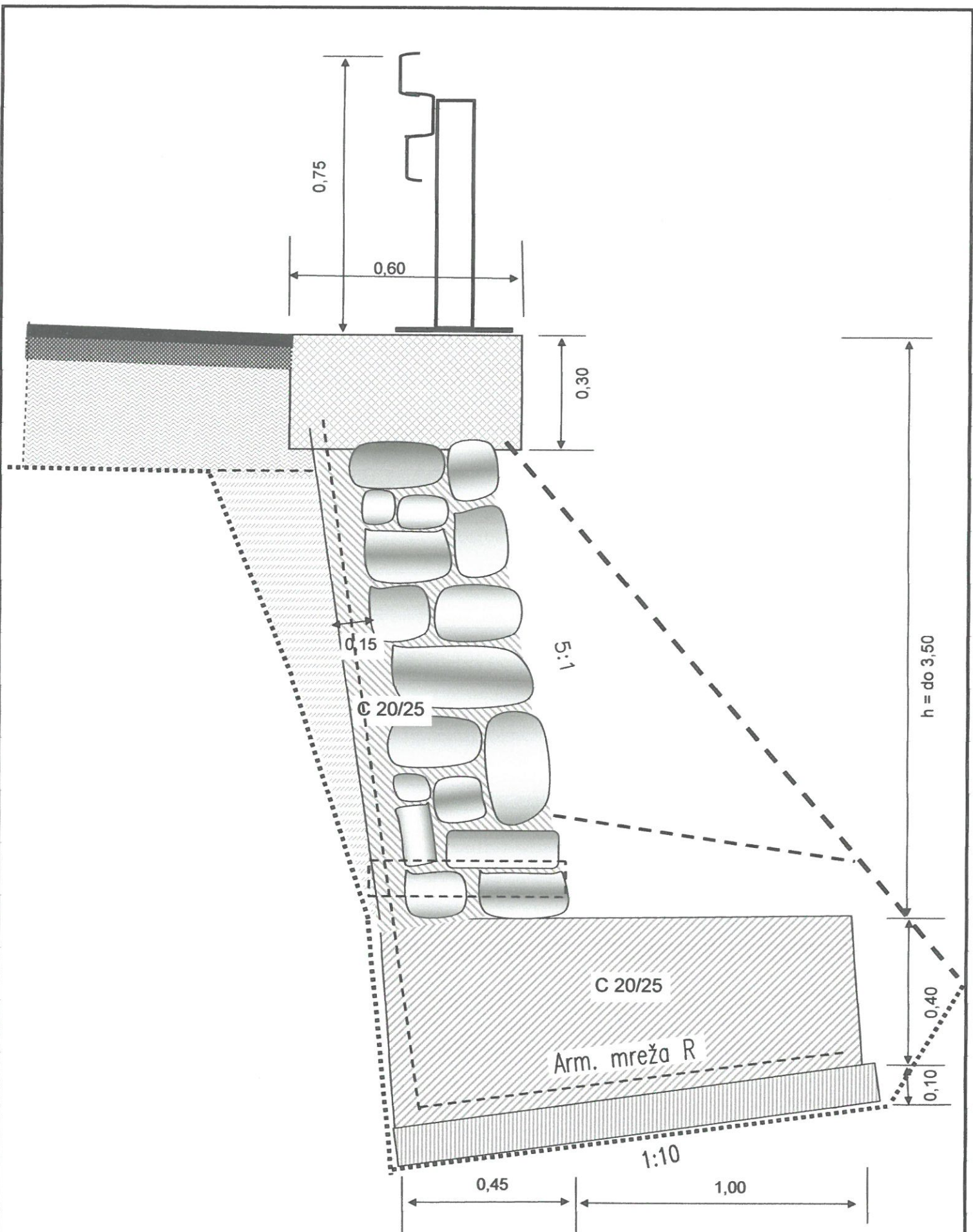
DETAJ ZA IZVEDBO KAMNITO-AB ZLOŽBE IZ PEŠČENJAKA Pri izvedbi del je potrebno detajl prilagoditbi geološkim razmeram.
