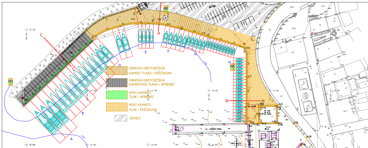
Načrt tlakovanja ribiškega pomola.
