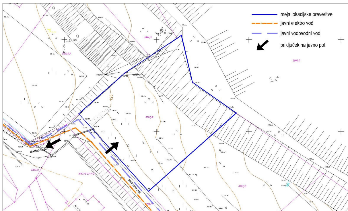
Slika št.6: prikaz komunalne opremljenosti območja (vir: geodetski posnetek GGS Geo139)
