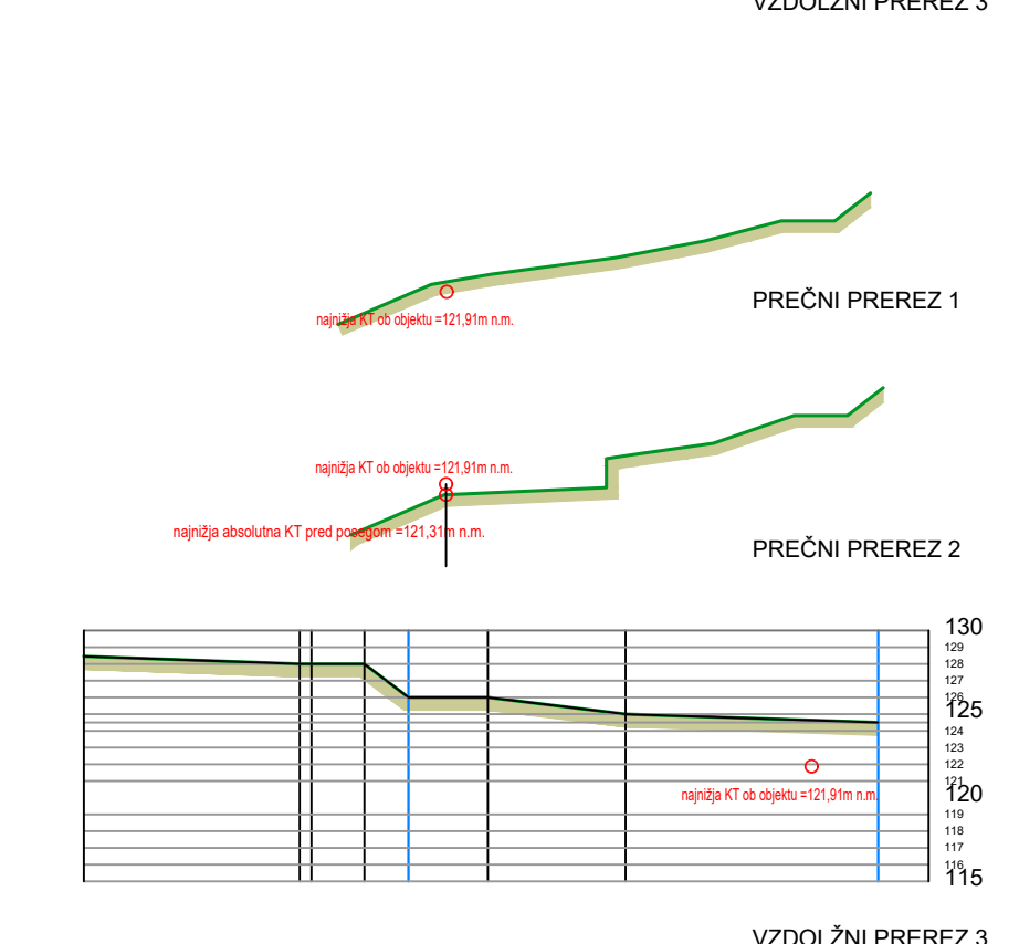
VZDOLŽNI PREREZ 3
