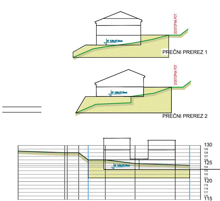
VZDOLŽNI PREREZ 3
