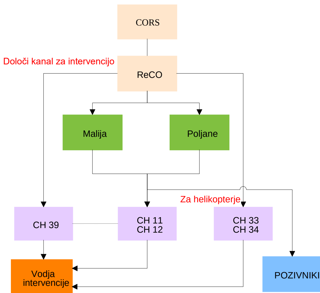
Slika 7: Načrt uporabe zvez med intervencijami
