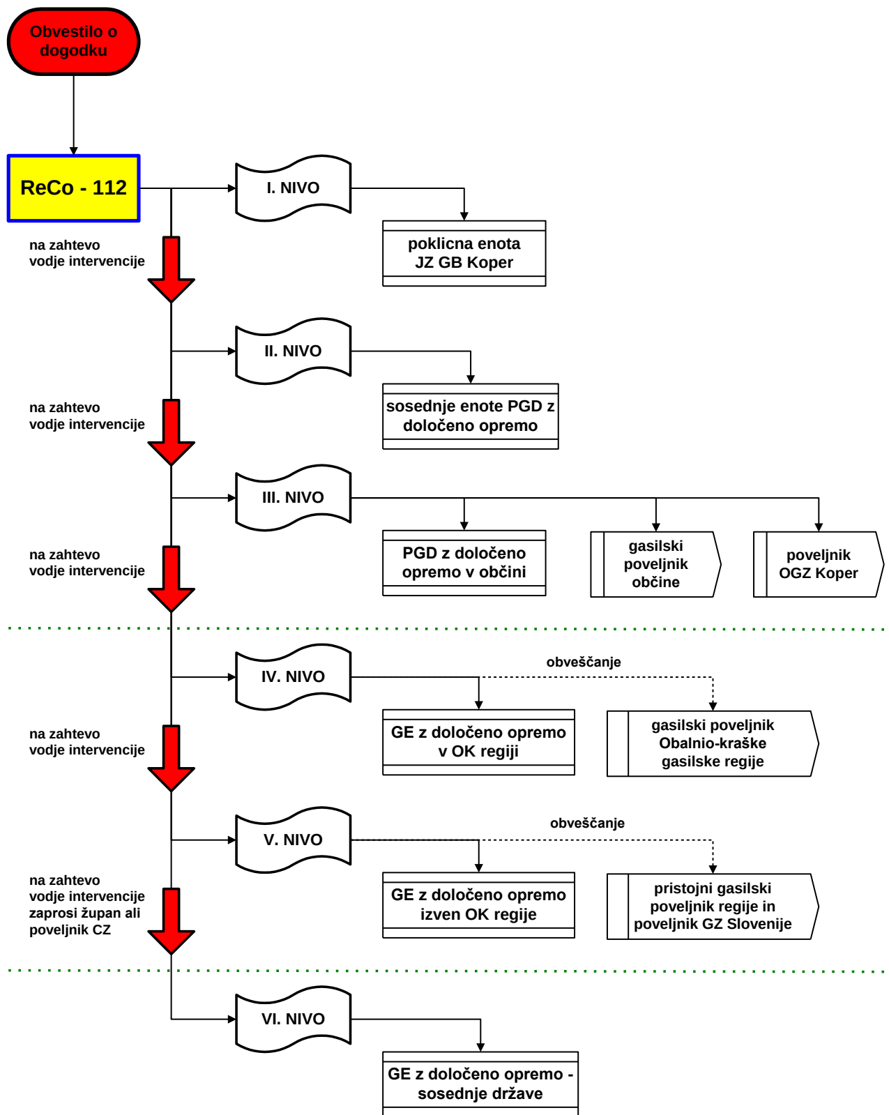
Slika4: Shema aktiviranja gasilskih enot pri tehničnih nesrečah, nesrečah v prometu in nesrečah z nevarnimi snovmi
