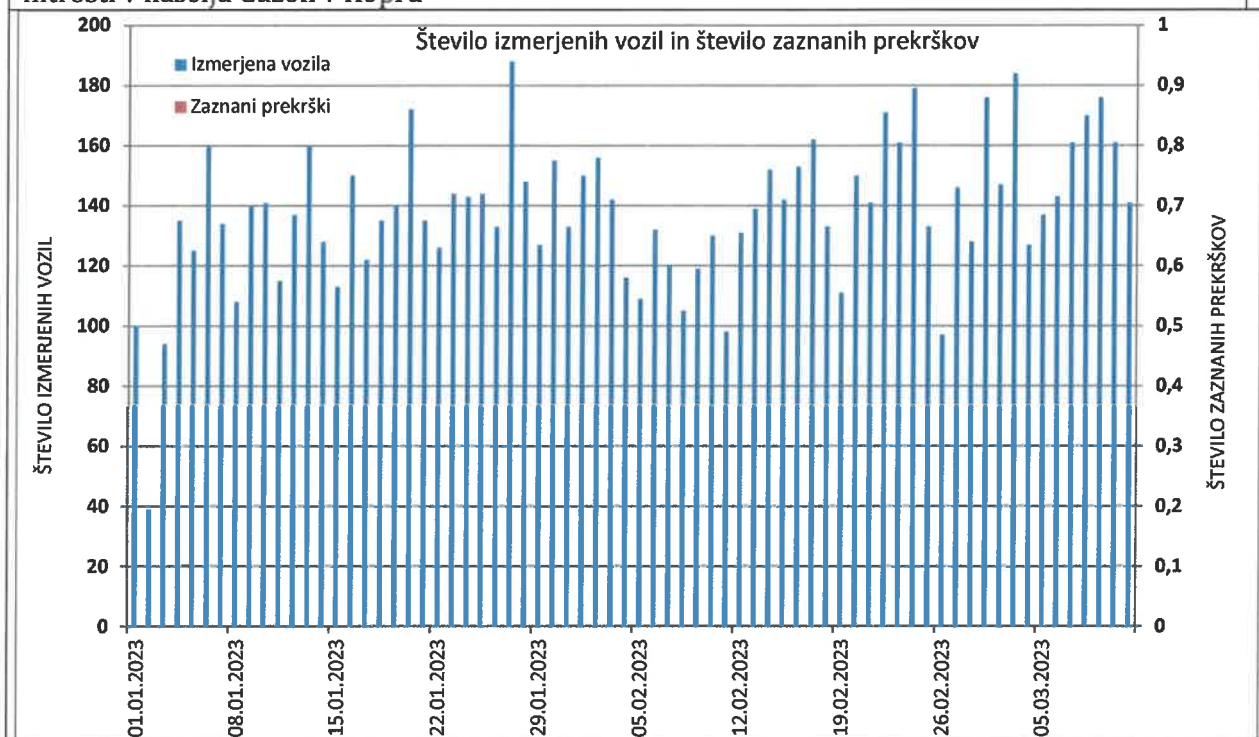
Prikaz števila izmerjenih vozil preko oba senzorja in število zaznanih prekrškov merilnika hitrosti v naselju Gažon v Kopru
