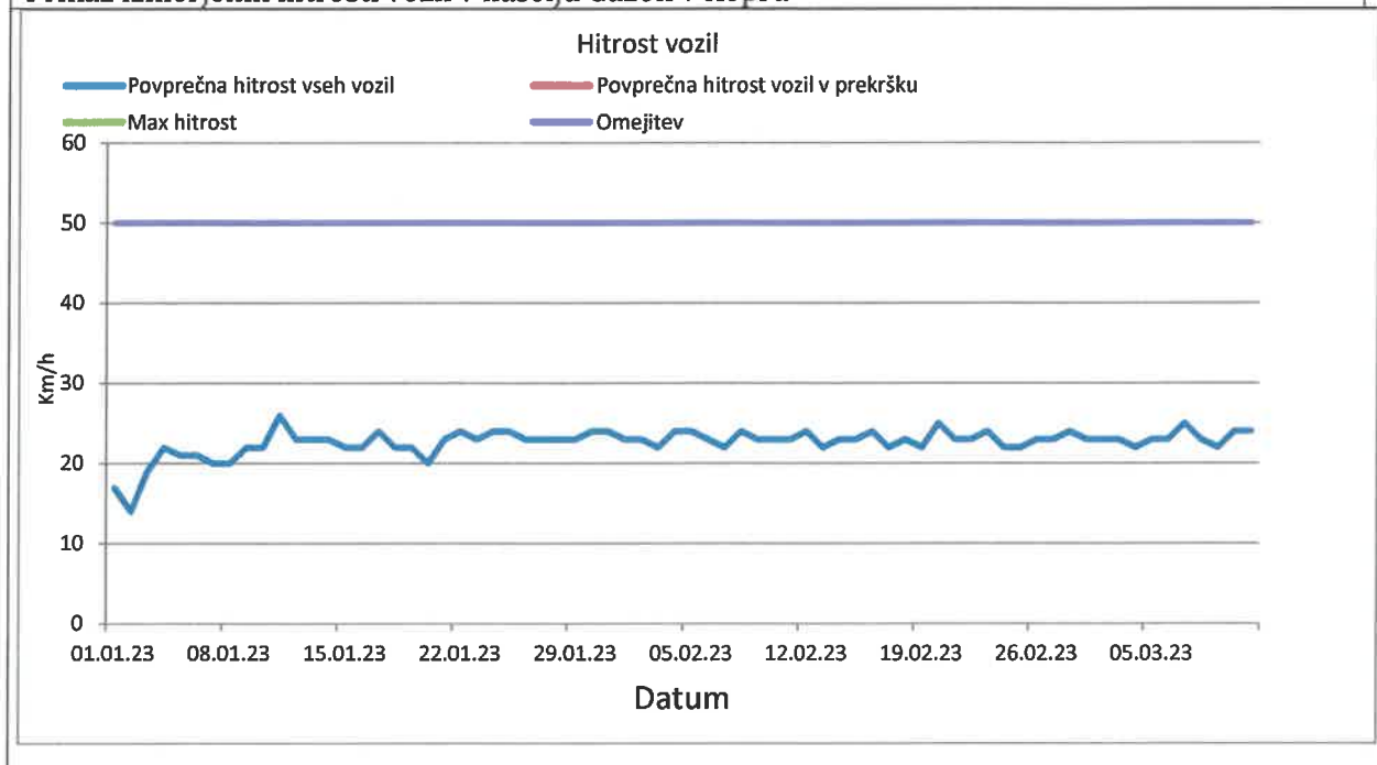
Prikaz izmerjenih hitrosti vozil v naselju Gažon v Kopru
